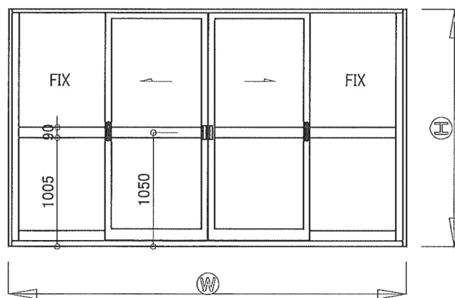
両袖FIX引分け戸
